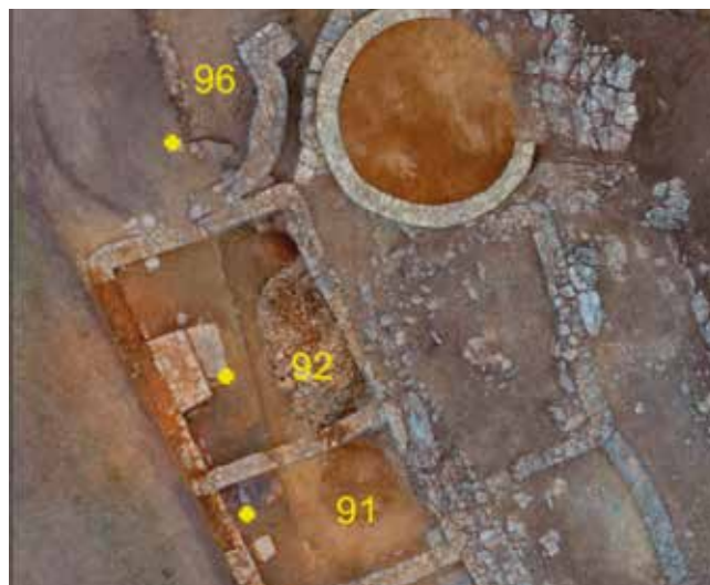
Fig. 20. Na fotografía móstrase cun punto amarelo o lugar onde se recolleron as mostras asociadas ós carbóns depositados sobre o chan e asociados ó derradeiro momento de ocupación da vivenda. As gráficas correspóndense cos datos das tres datacións.
