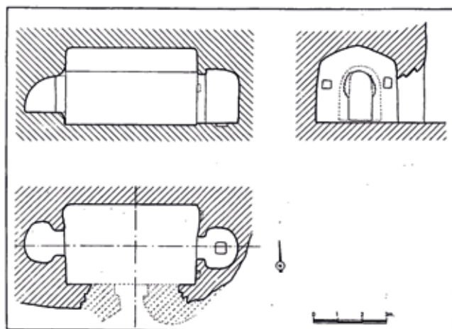
Fig. 35. Planta da igrexa rupestre de San Pedro de Tartalés de Cilla, en Burgos. Segundo L. Alberto Monreal e Jesús M. Monreal, tomado de Monreal Jimeno, L. A.: "Arquitectura religiosa de oquedades en los siglos anteriores al románico", en VII Semana de Estudios Medievales de Nájera , 1997, pp. 235-263.
